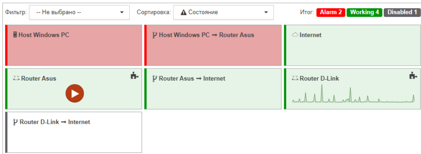
Рис. 8. Вид сетки
