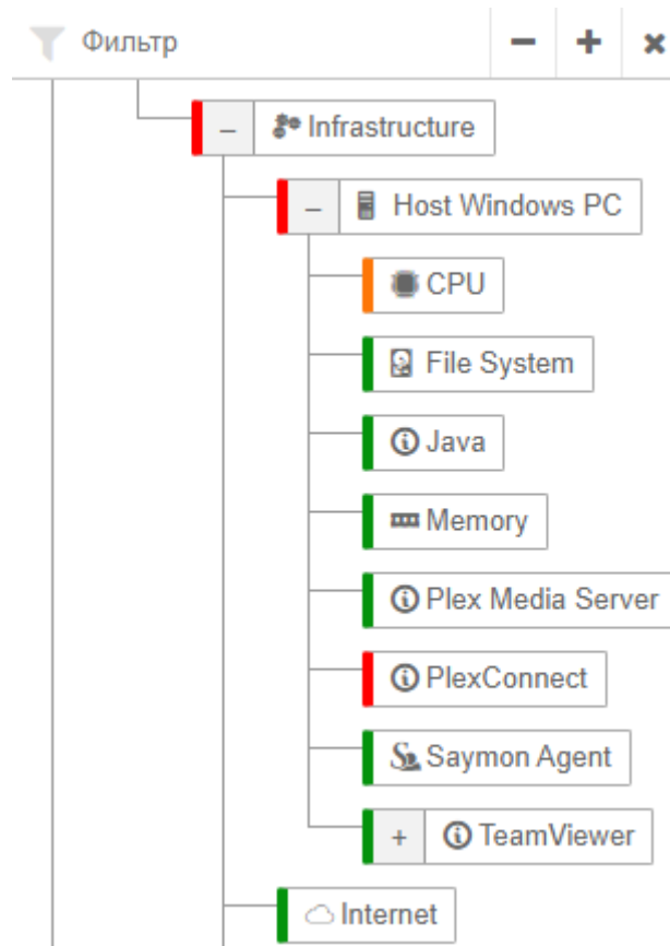
Рис. 20. Панель навигации
