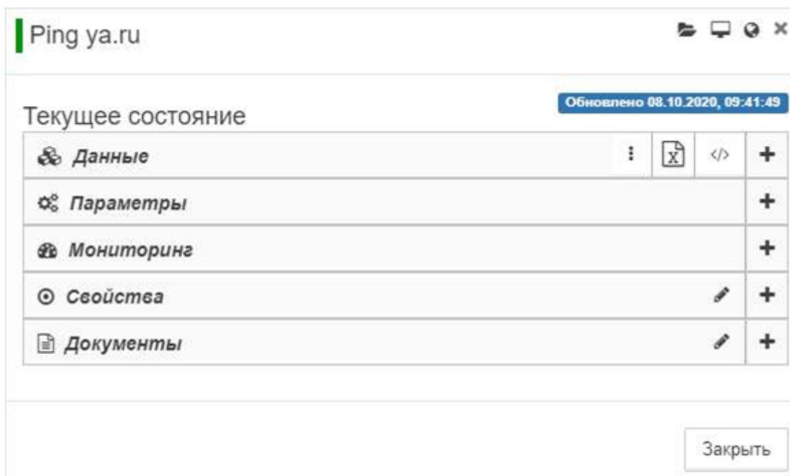
Рис. 12. Окно информации
