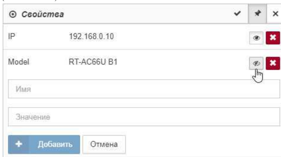
Рис. 4.10.2.2. Настройка отображения свойств в подписи к объекту
