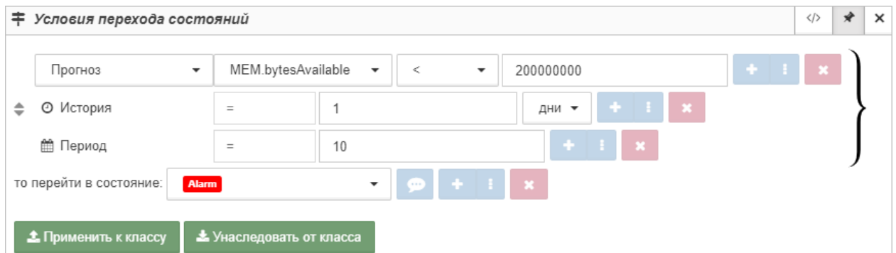
Рис. 4.4.3.2. Пример правила для прогнозирования значения метрики
