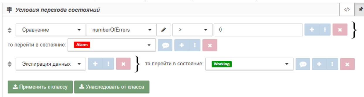
Рис. 4.2.2.4. Пример настройки условия с типом "Экспирация данных"
