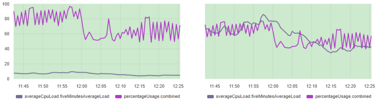
Рис. 4.5.7.6. Масштабирование значений на мультиграфике
