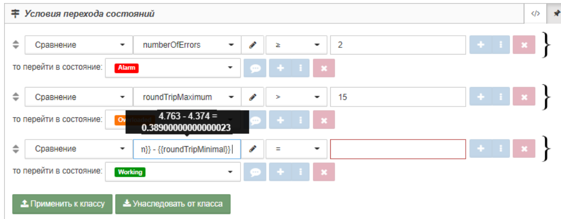
Рис. 4.2.2.3. Ввод математической формулы
