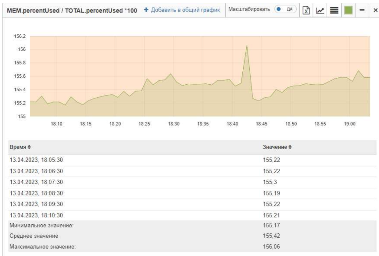
Рис. 4.5.7.8. Пример графика на основе математической формулы
