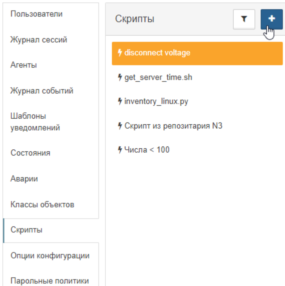
Рис. 4.11.10.1. Репозитарий скриптов
