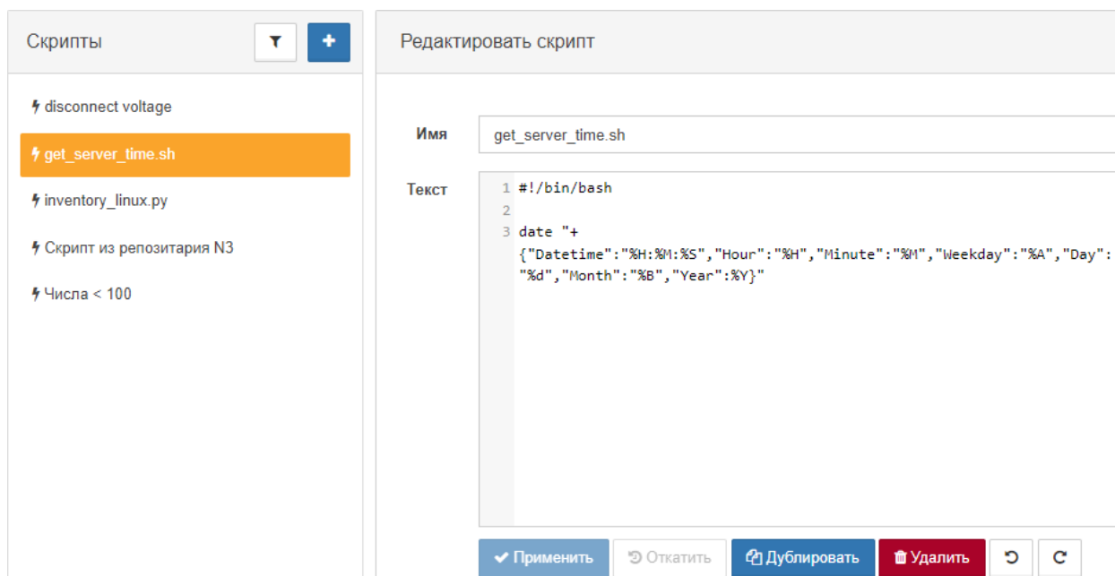
Рис. 4.11.10.2. Редактирование скриптов
