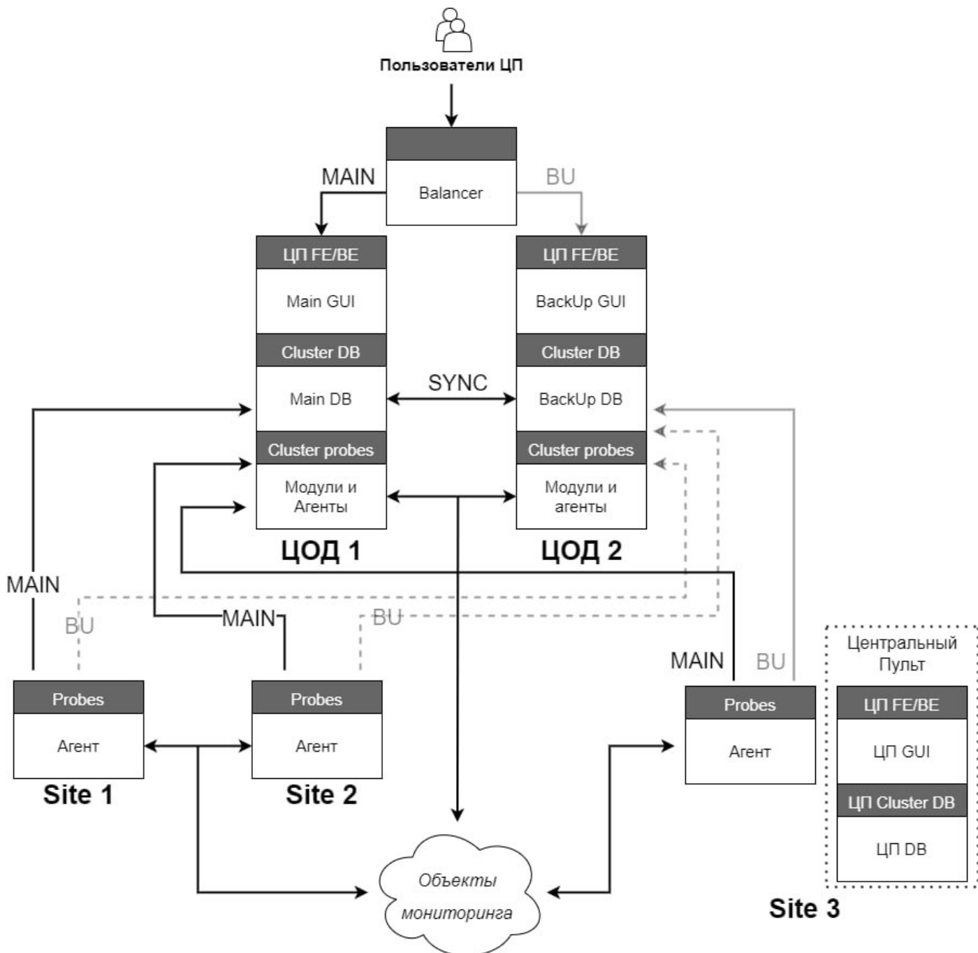
Рис. 2. Отказоустойчивое исполнение системы
